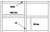
TYPE 1 ระยะแป (SPAN): 139.2 เซนติเมตร ระยะจันทัน (RAFTER): 120 เซนติเมตร
