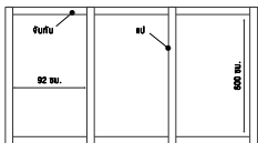
TYPE 2 ระยะแป (SPAN): 92 เซนติเมตร ระยะจันทัน (RAFTER): 600 เซนติเมตร
